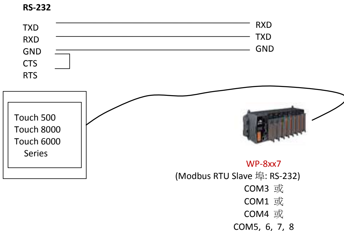
接線圖
