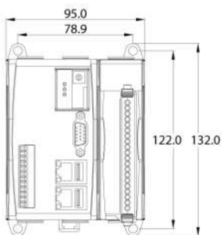
前視圖
