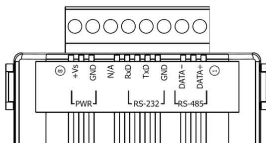
圖 2-3、IR-712 可卸式螺絲端子
