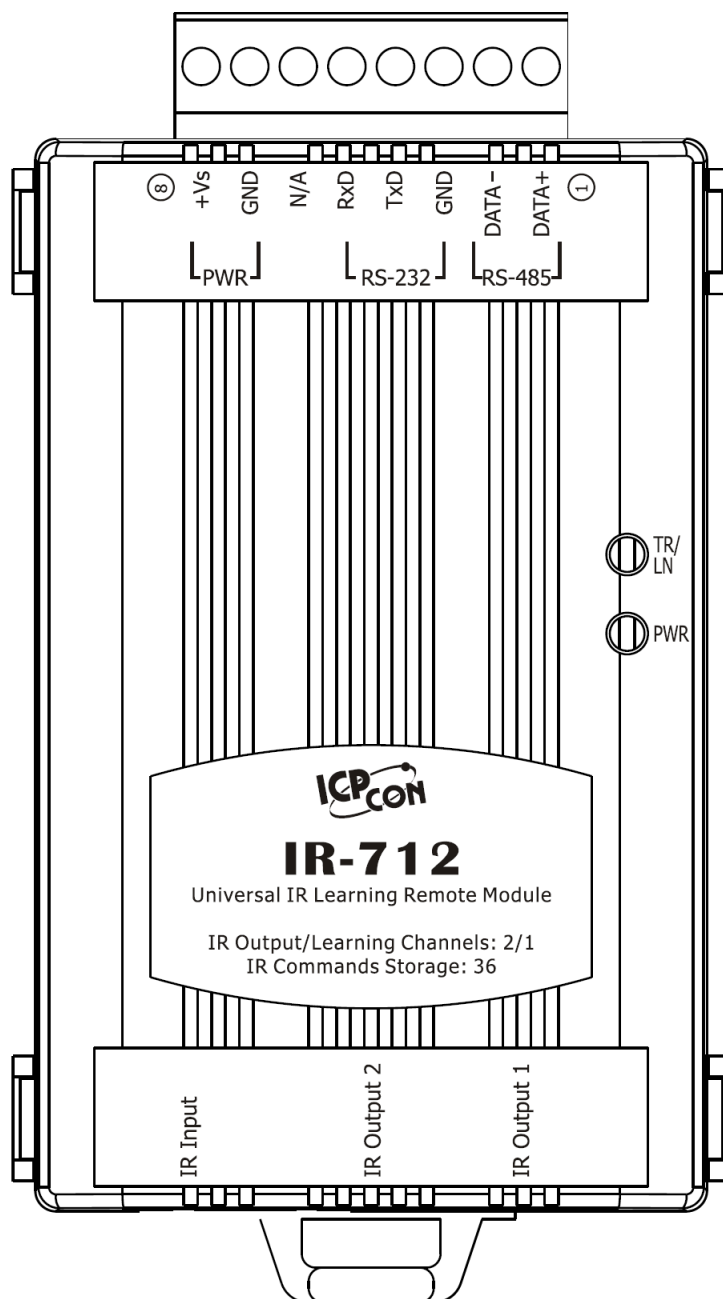
圖 2-1、IR-712 產品前方外觀
