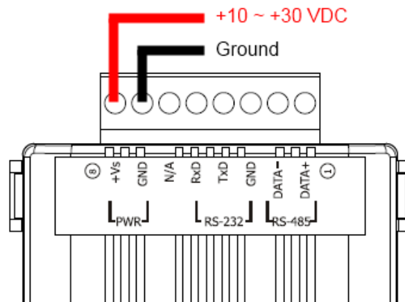
圖 2-10、電源接線圖
