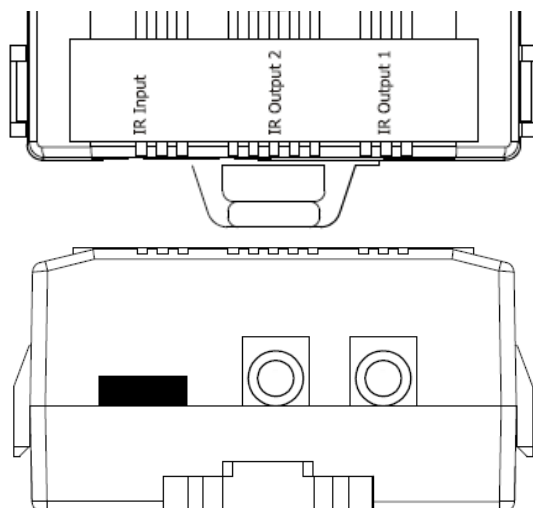
圖 2-2、IR 輸出 3.5 mm 音源插座與學習輸入孔 (前視圖/下視圖)
