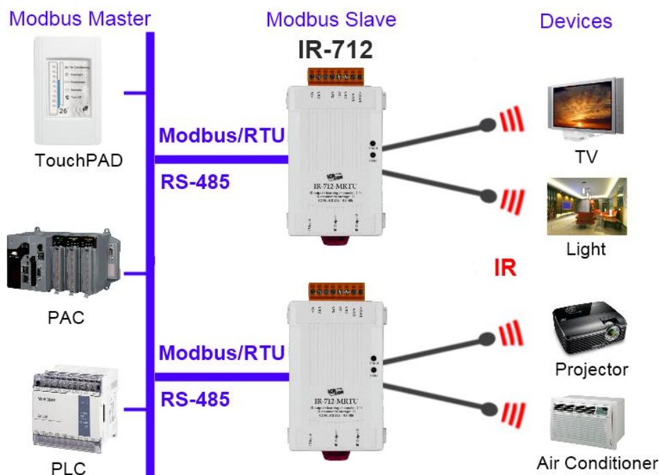
圖 1-1、IR-712 之 RS-232/RS-485 介面應用架構
