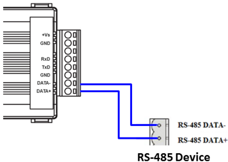
圖 2-7、RS-485 連線
