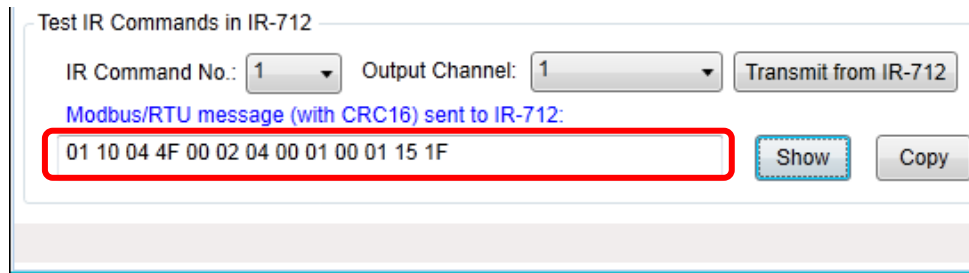
圖 4-8、測試 IR-712 內存之 IR 命令
