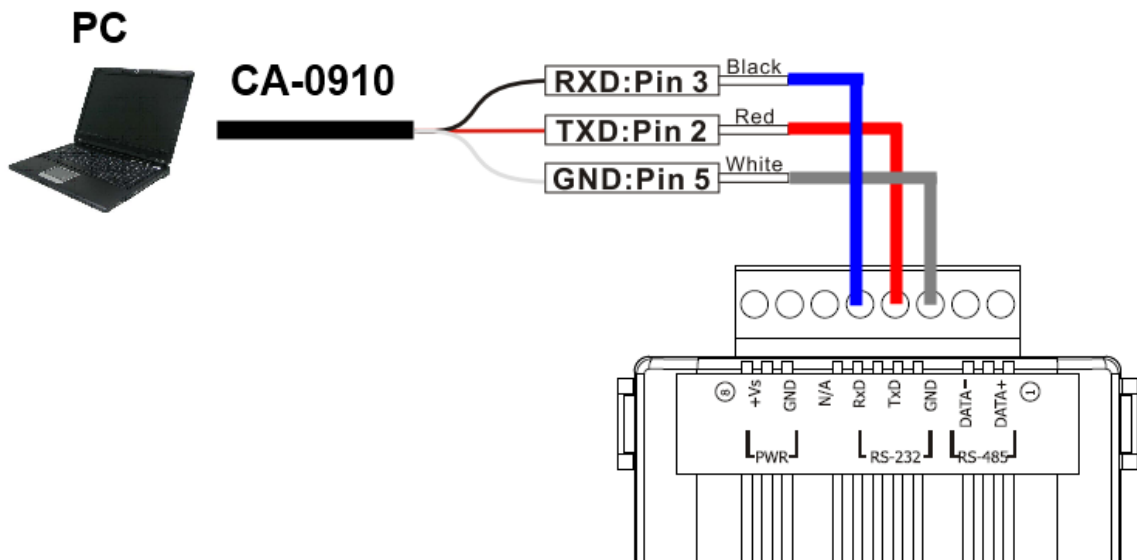
圖 2-6、CA-0910 傳輸線與 IR-712 接線腳位
