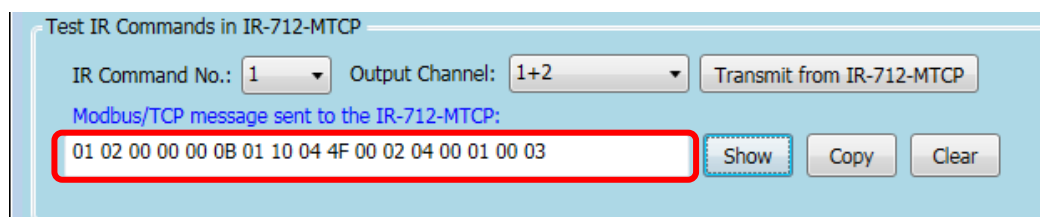
圖 4-8、測試 IR-712-MTCP 內存之 IR 命令
