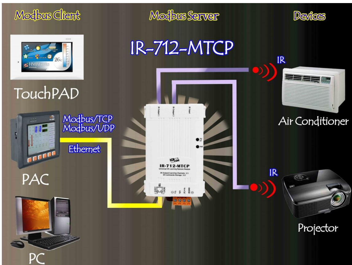
圖 1-1、IR-712-MTCP 基本應用架構
