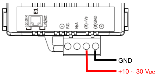
圖 2-6、電源接線圖
