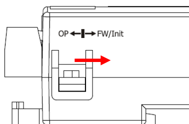
圖 2-8、指撥開關撥至 FW 位置
