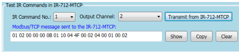
圖 3-15、測試 IR-712-MTCP 內存之 IR 命令
