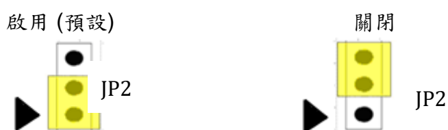
圖 2-7、看門狗計時器 JP2 跳線位置
