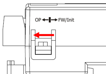
圖 2-9、指撥開關撥至 OP 位置
