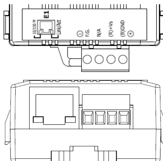
圖 2-3、IR-712-MTCP 端子台
