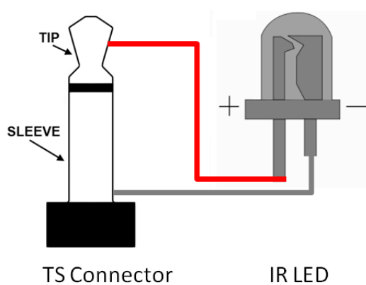
圖 2-5、TS 接頭連接 IR LED
