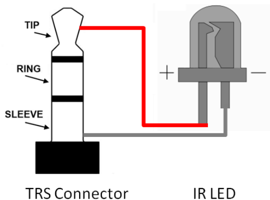
圖 2-4、TRS 接頭連接 IR LED
