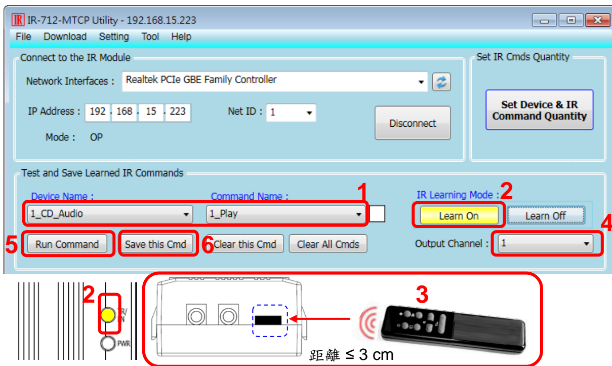
圖 4-6、學習 IR 命令步驟
