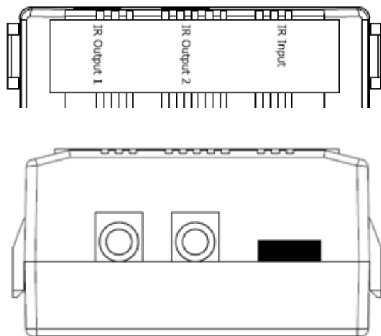
圖 2-2、IR 輸出 3.5 mm 音源插座與學習輸入孔
