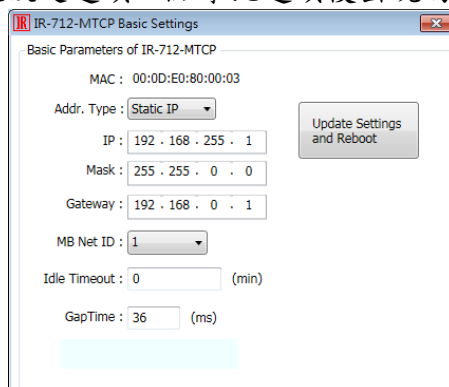
圖 3-5、IR-712-MTCP 基本參數設定視窗
