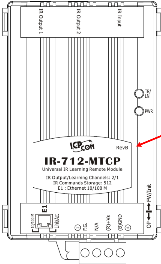
Fig.1-1 IR-712-MTCP front
