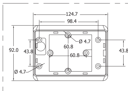
牆壁安裝
