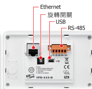
TPD-433-H 後視圖
