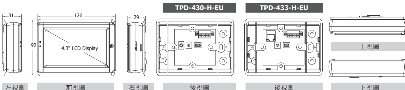
左視圖
