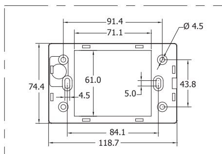
牆壁安裝
