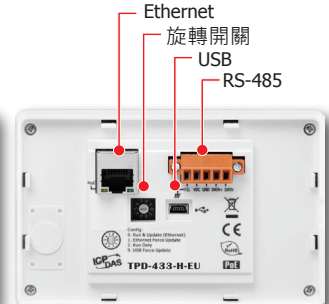
TPD-433-H-EU 後視圖
