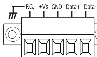
TPD-430-H 後視圖
