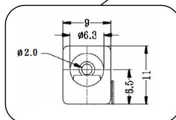
上視圖
