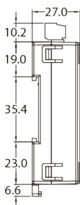
左側視圖
