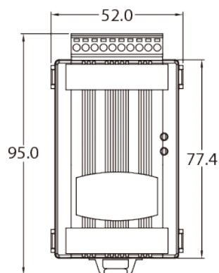
前視圖
