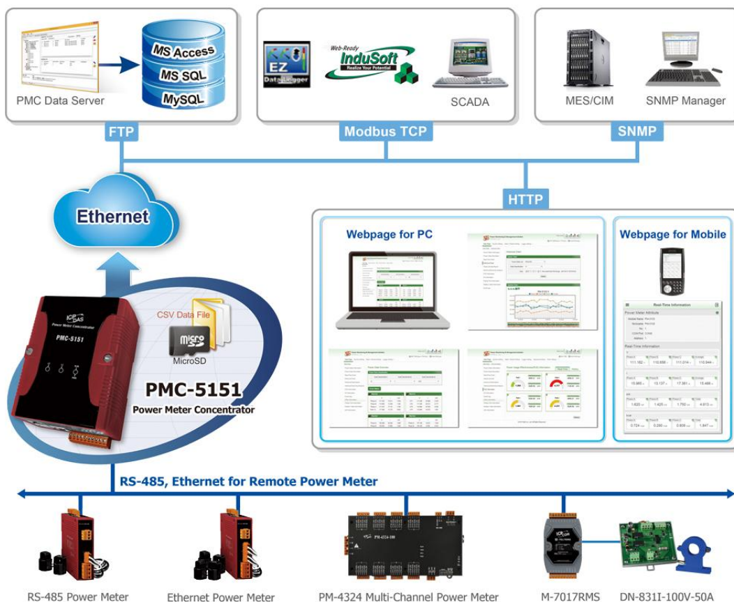
圖1-1: 系統架構圖
