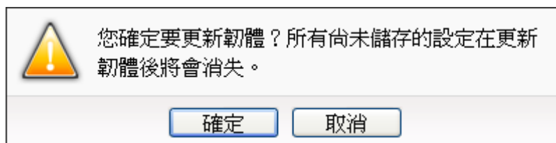
圖6-35: 韌體更新(4)
