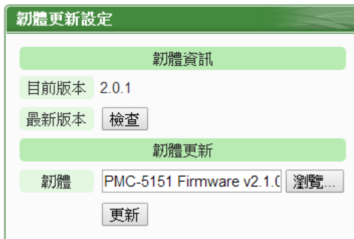
圖6-34: 韌體更新(3)
