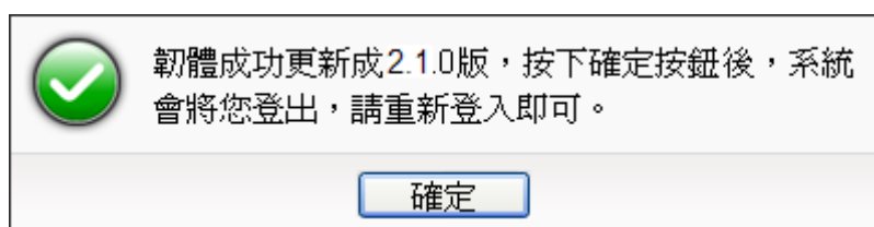
圖6-37: 韌體更新(6)
