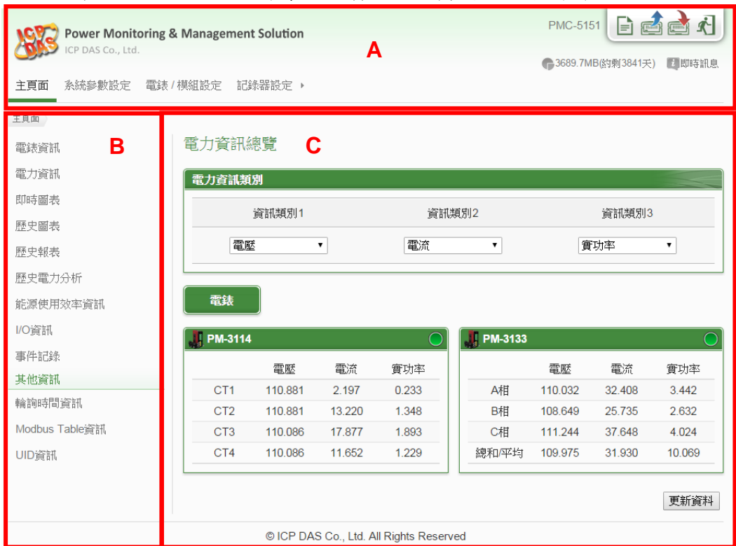
圖4-1: 系統首頁
