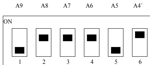
SW1 : BASE ADDRESS (☑): 預設基準位址 0x220
