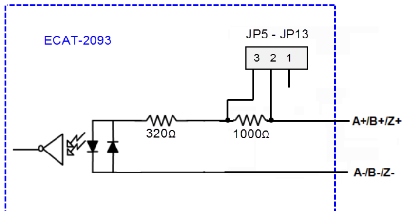
圖 7: 編碼器通道電路
