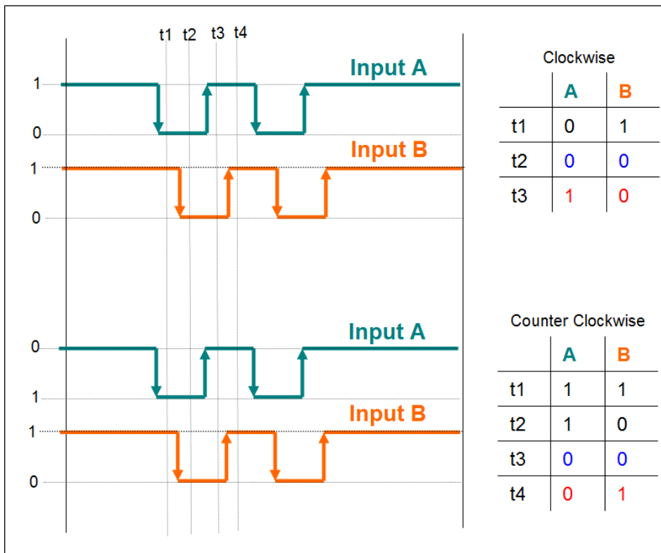
圖 26: 輸入信號"A"極性改變 反轉計數方向
