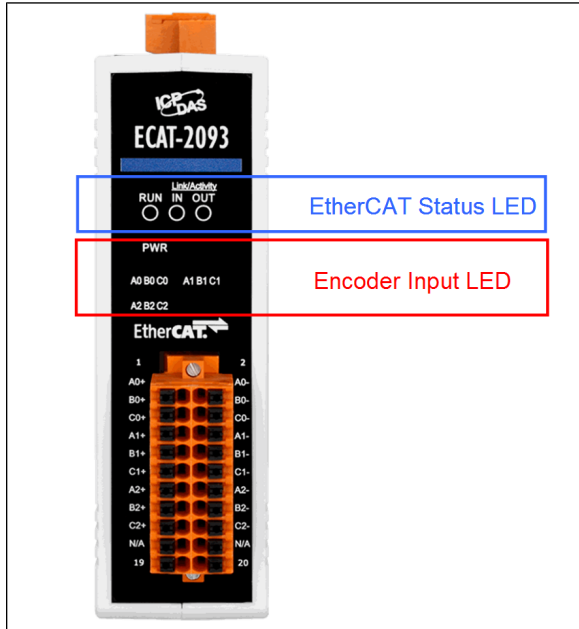
圖 3: ECAT-2093 LEDs
