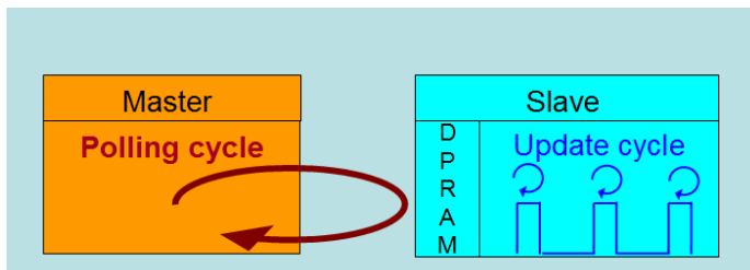
圖 15: DC 同步模式下的主站與從站週期
