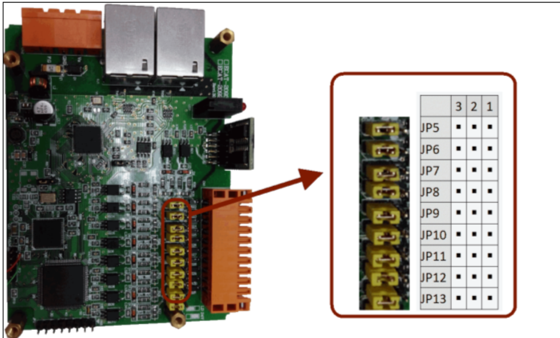
圖 9: 跨接器位置
