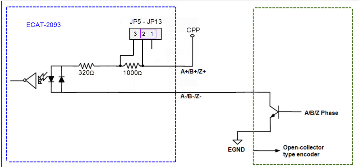
圖 8: 開路集極接線圖
