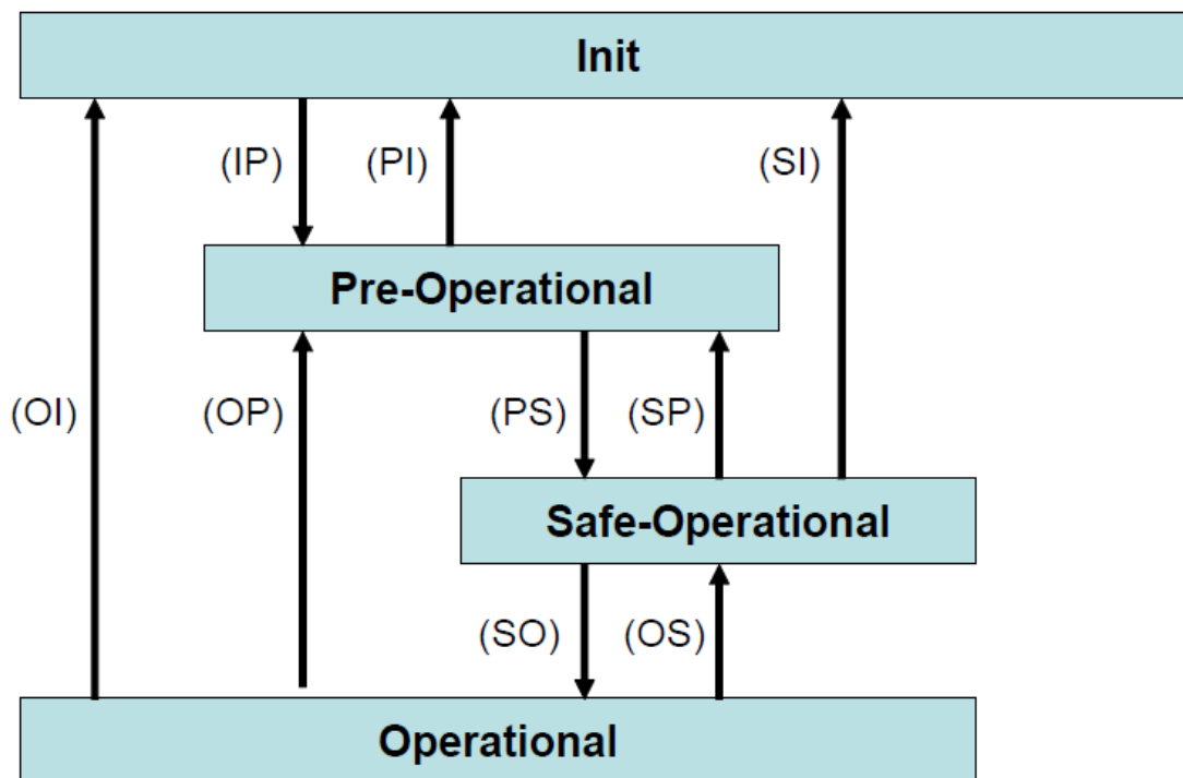
圖 10: EtherCAT 狀態機
