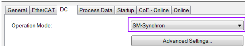
圖 14: SM-Synchron 模式選擇
