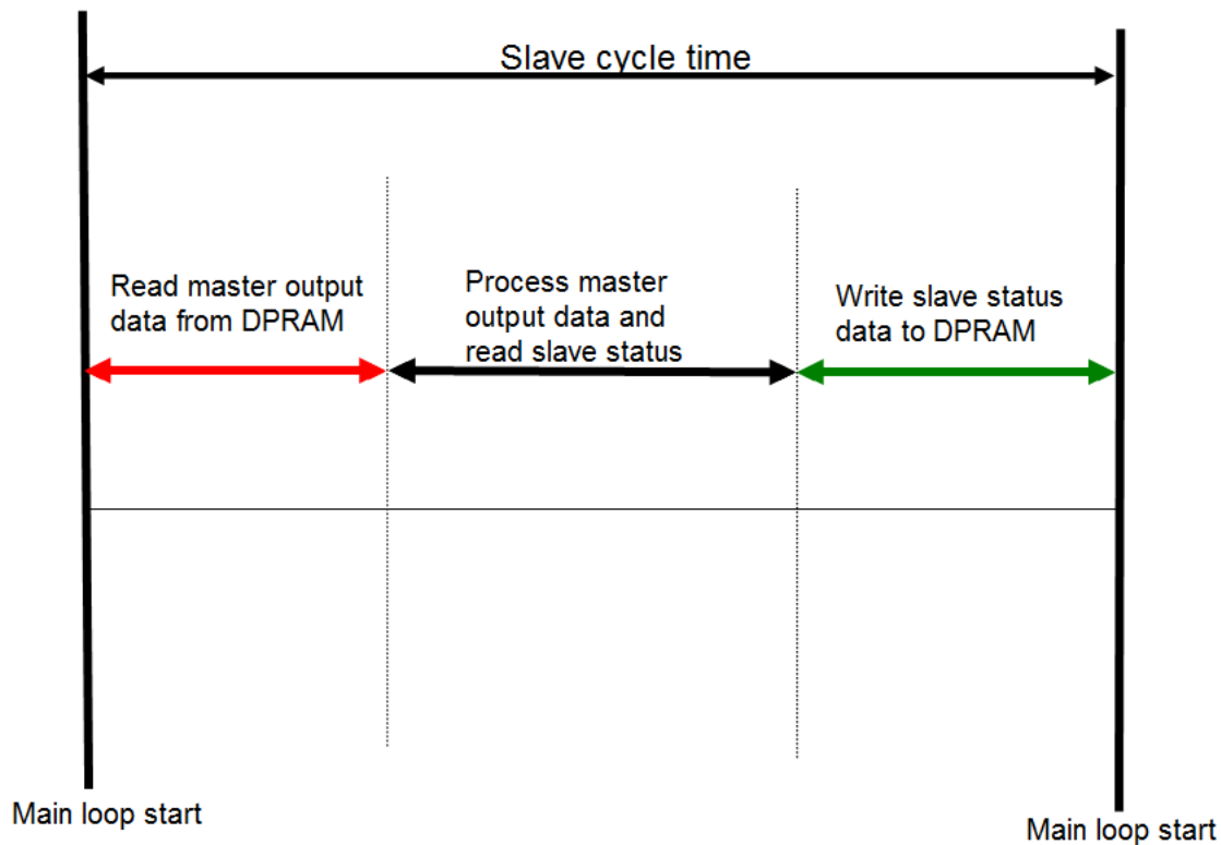
圖 12: 自由運行模式下的從站處理序列
