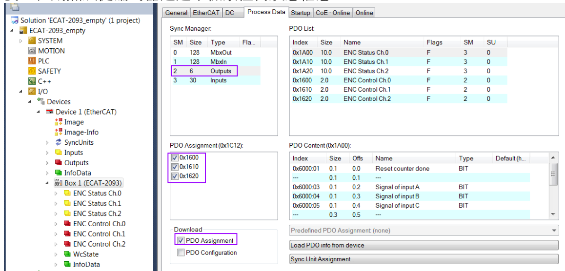
圖 21: Predefined PDO assignment 選項
