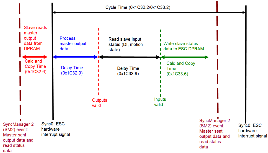
圖 16: DC 同步模式下的內部從站處理序列
