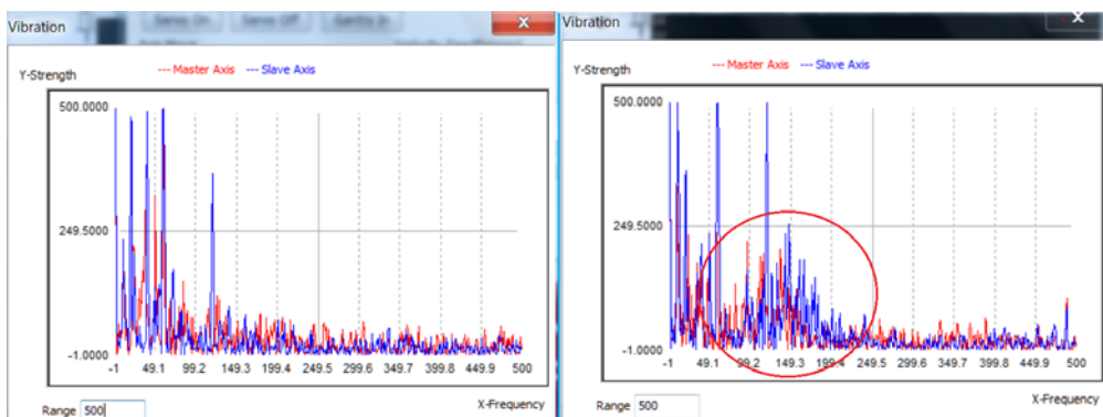
KP過大，開始有震盪，如果再將 KP 加大，可能導致位置發散!
