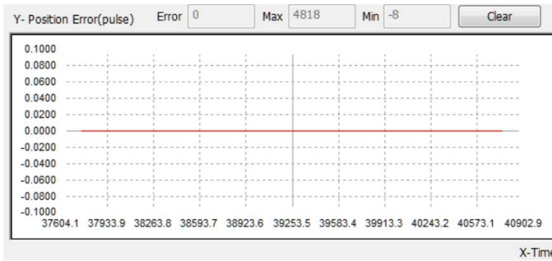
● 位置誤差顯示框，顯示主軸與從軸的位置誤差(單位: pulse)，Error 為當前誤差，Max 為最大誤差，Min 為最小誤差，按下 Clear 可以清除 Max 與 Min 的數值。
