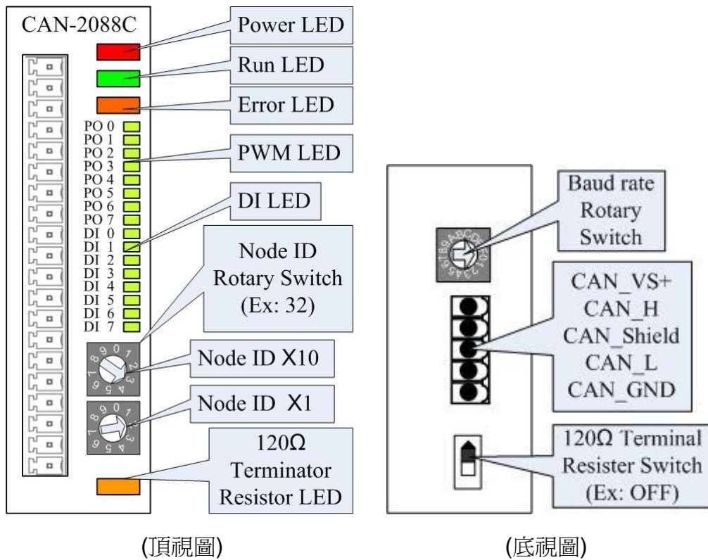
圖 2-1 CAN-2088C LED 規劃圖、端子與旋鈕開關
