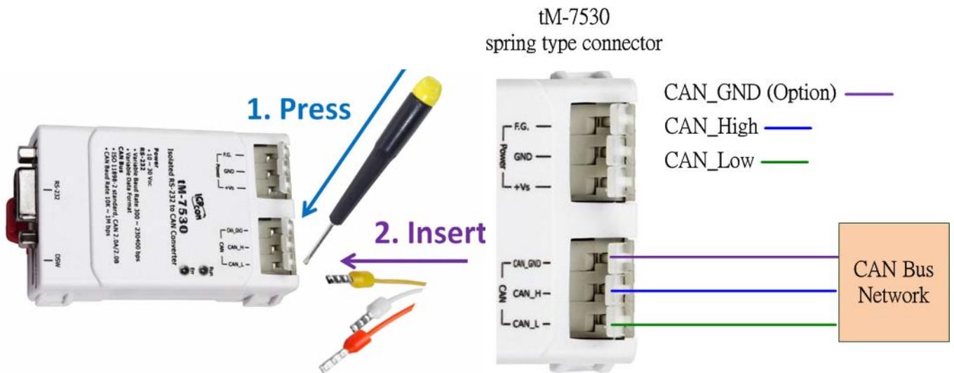
圖：tM-7530 CAN 總線接線方式
