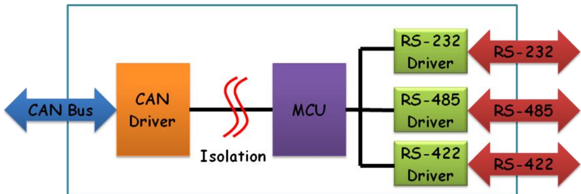
圖：I-7530A 硬體方塊圖
