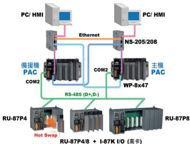
Hot Swap! RU-87P4/8 + I-87K I/O (高卡)
