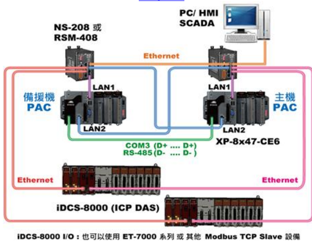
iDCS-8000 I/O : 也可以使用 ET-7000 系列 或其他 Modbus TCP Slave 設備
