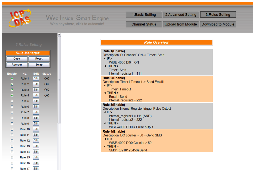
圖 6-29：所有規則的描述總表
