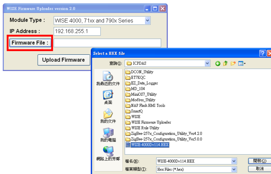
圖 11-12：選擇韌體更新檔
