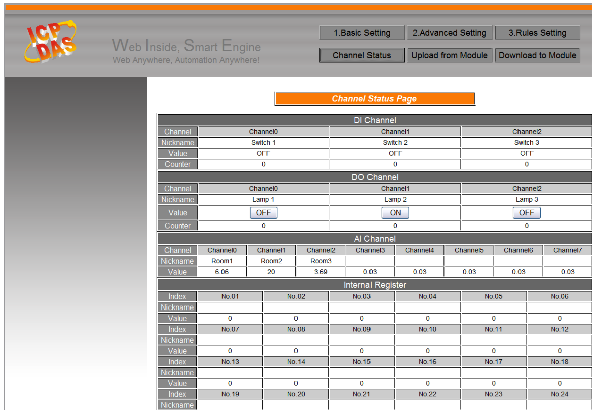
圖 9-1：Channel Status 的頁面
