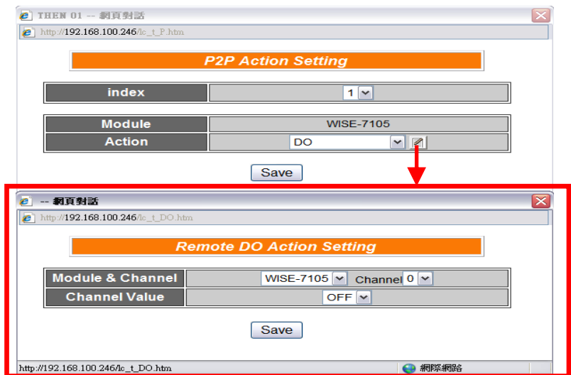
圖 6-26：P2P 的動作細項設定頁面
