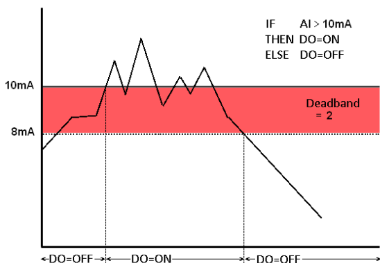
圖 10-10：AI Deadband 示意圖(作用於大於條件)
