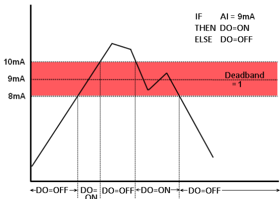
圖 10-12：AI Deadband 示意圖(作用於等於條件)
