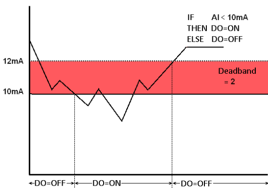
圖 10-11：AI Deadband 示意圖(作用於小於條件)
