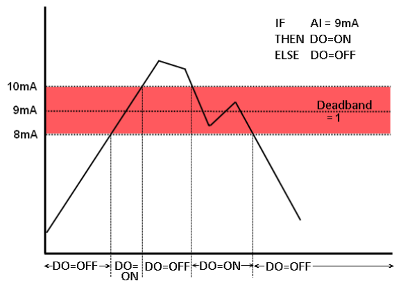
图 10-11: AI Deadband 示意图(作用于等于条件)
