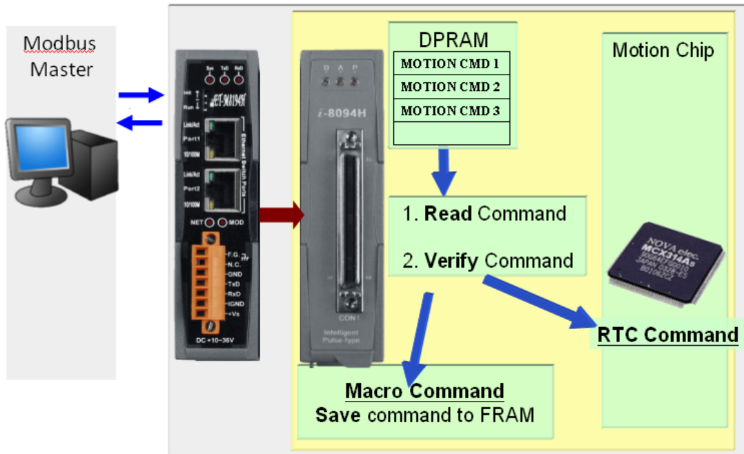
圖 2 安裝於插槽 1 的 i-8094H 模組
