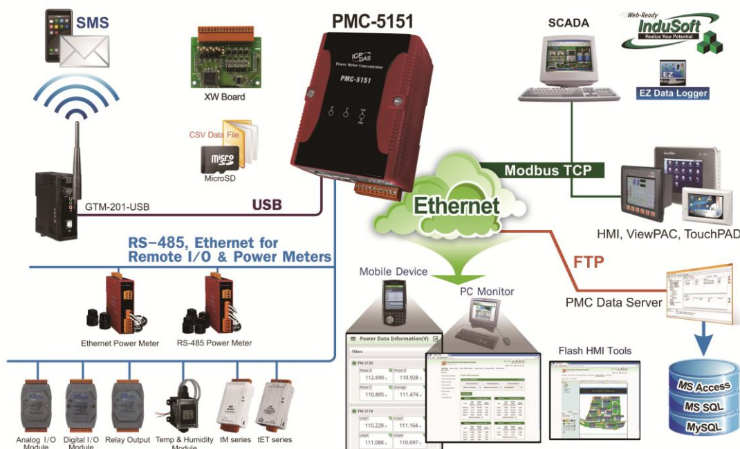
图1-1: PMC-5151 系统架构图
