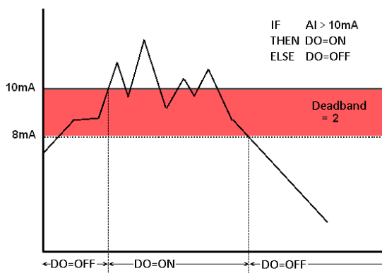
图7-22: AI Deadband 示意图(作用于大于条件)
