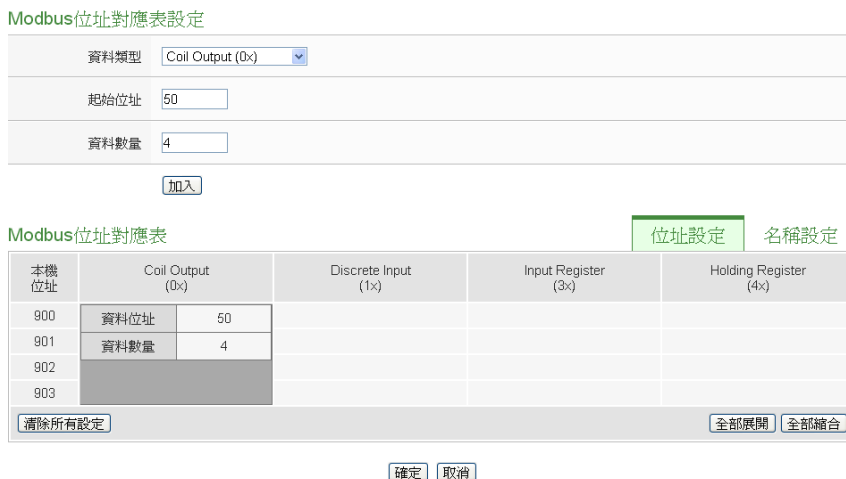
图7-44: Modbus RTU 模块 Coil Output 数据设置页面范例
