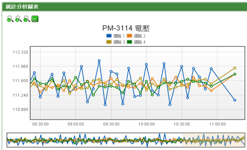
图5-17: PM-3114 历史趋势图
