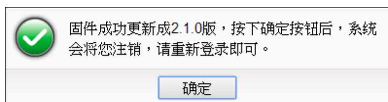
图6-37: 硬件更新(6)
