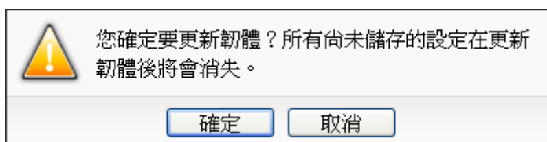
图6-35: 硬件更新(4)
