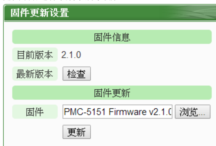
图6-34: 硬件更新(3)
