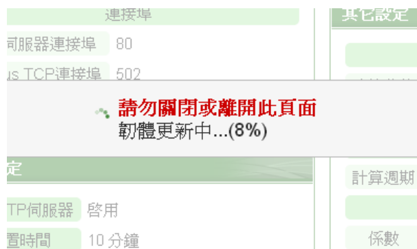
图6-36: 硬件更新(5)
