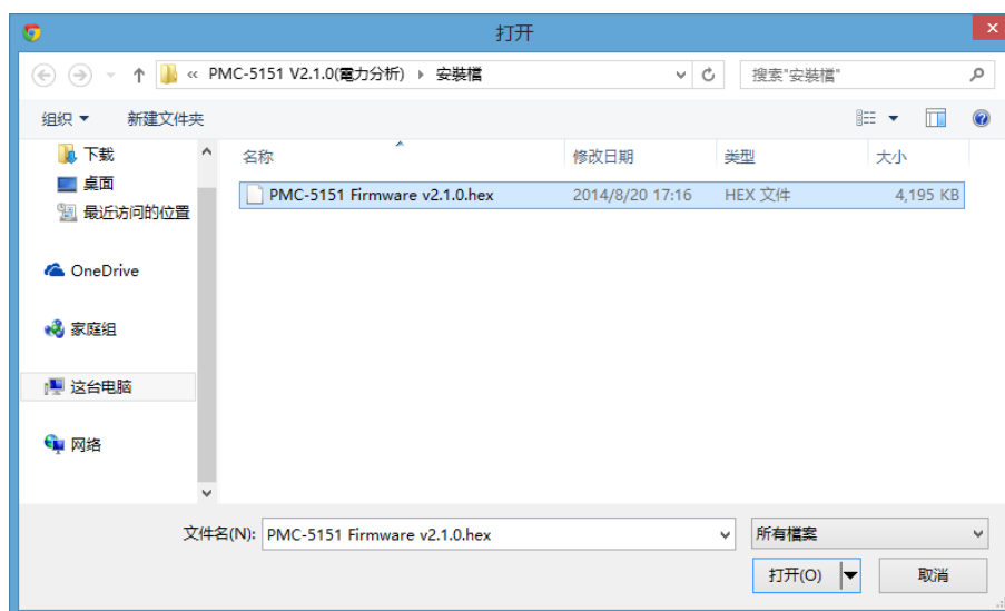
图6-33: 硬件更新(2)
