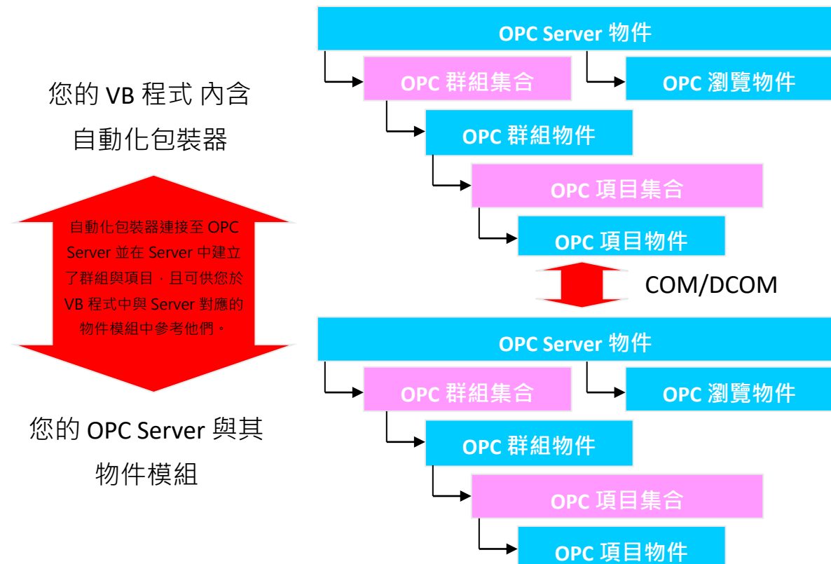
圖 5-1-2. 於 COM/DCOM 機制下 OPC Server 物件的架構
